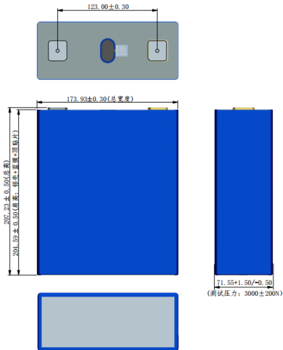
Figure 7 电池尺寸 /mm
