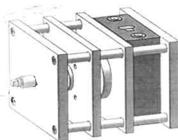
Fig. 5 Diagram of cell with swelling force clamp 图 5 电池上膨胀力夹具图
